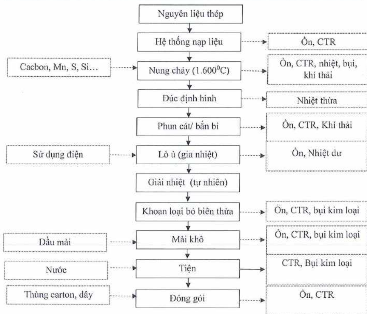
Hình 1-1 Quy trình công nghệ sản xuất
