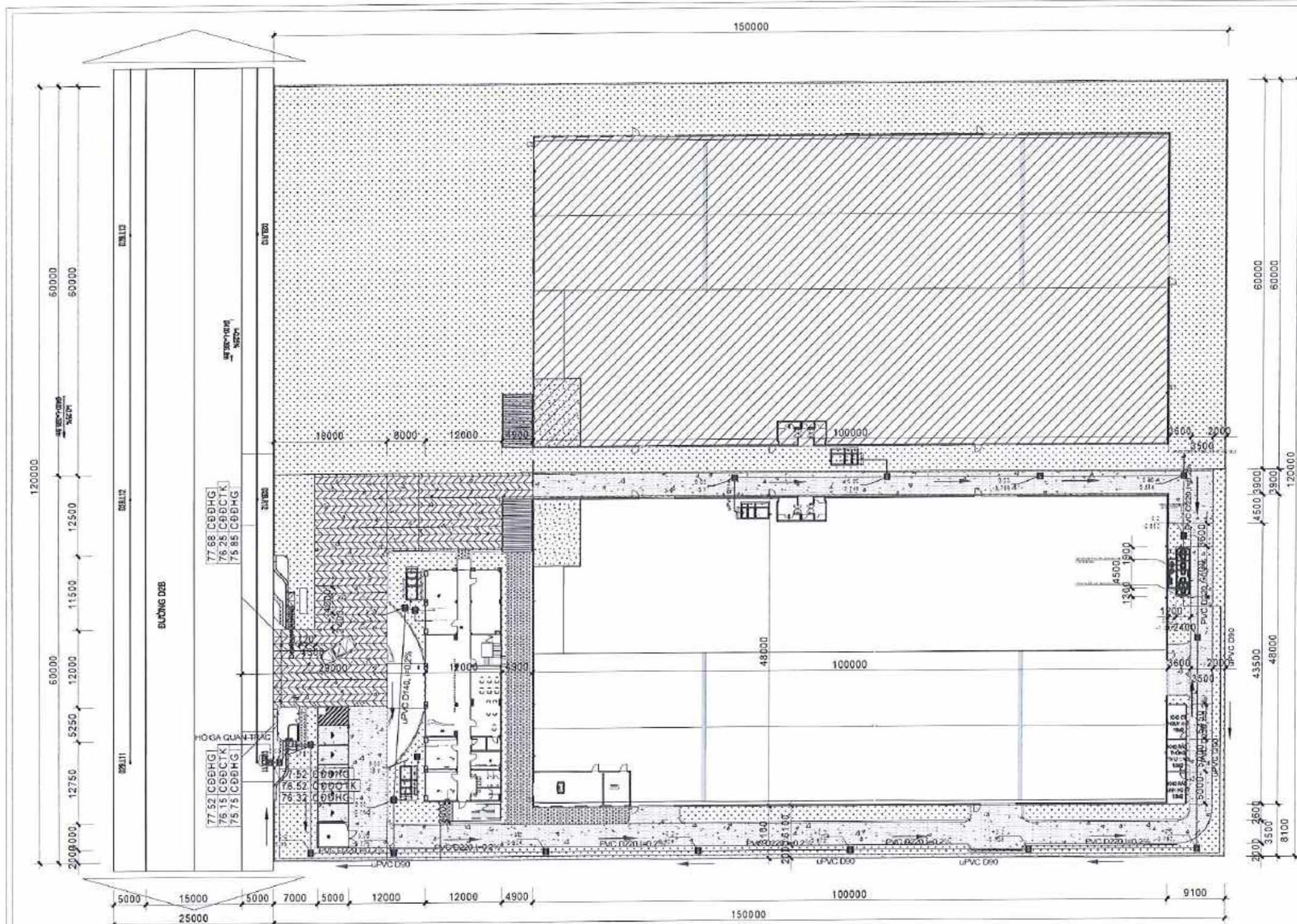
TỔNG MẶT BẰNG THOÁT NƯỚC THẢI TỶ LỆ 1/500
