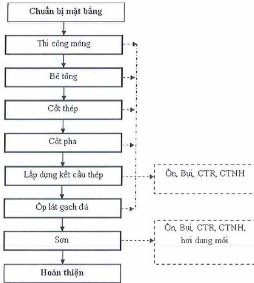
Hình 1-5 Quy trình thi công xây dựng các công trình.
