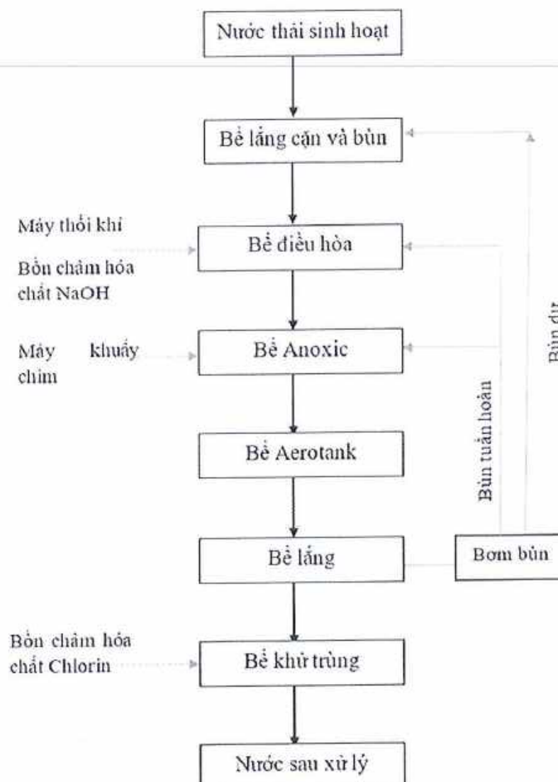
Hình 4-6 Sơ đồ xử lý nước thải tập trung tại Dự án
