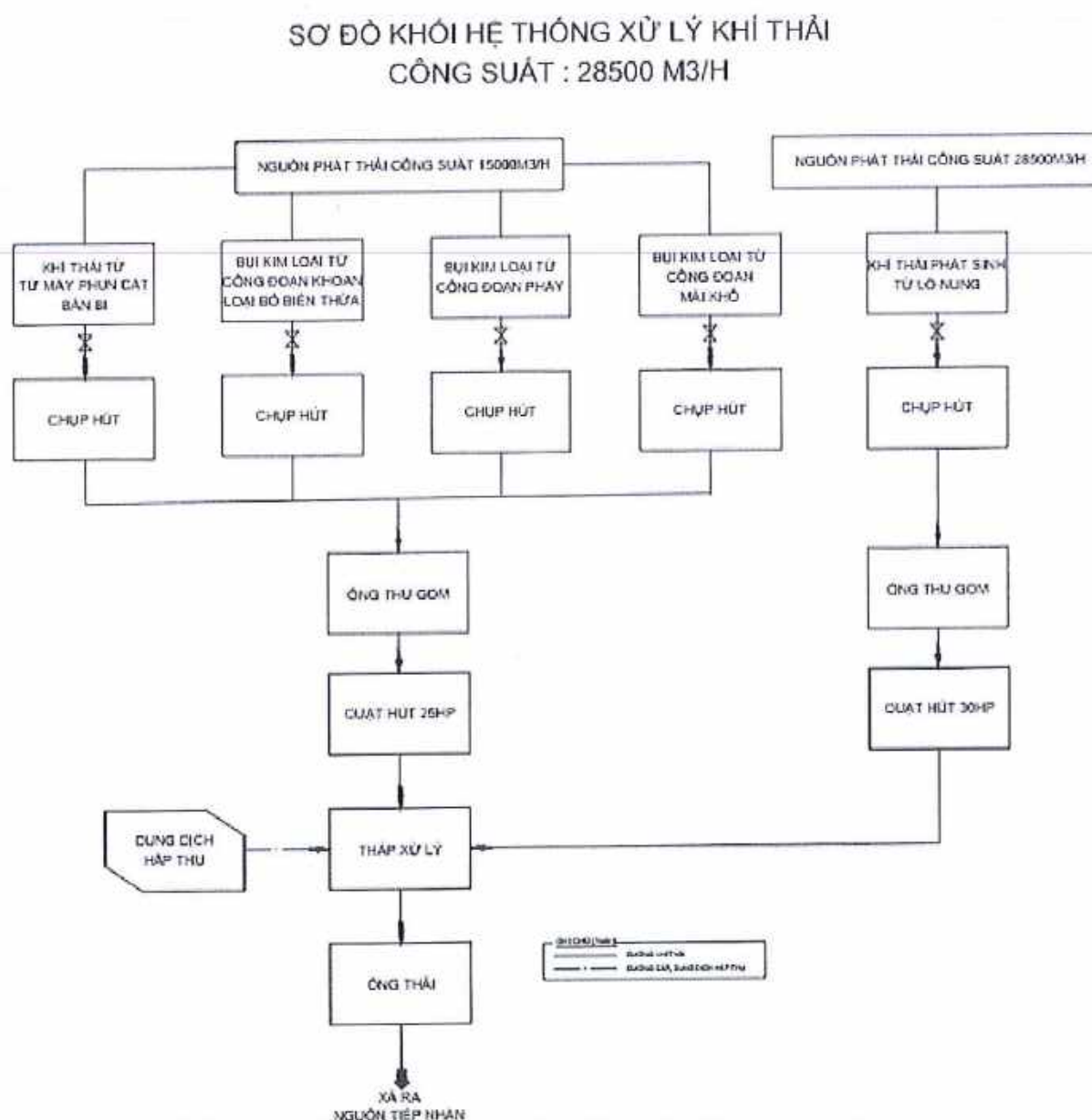
Hình 4-7 Sơ đồ thu gom xử lý bụi khí thải công suất 28.500 m 3 /giờ
