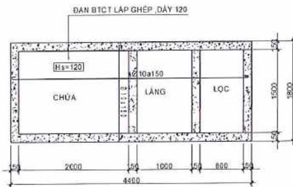
MẶT BẰNG BỐ TRÍ THÉP BÀN NÁP TỶ LỆ 1/50
