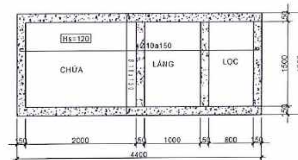
MẶT BẰNG BỐ TRÍ THÉP BÀN ĐÁY TỶ LỆ 1/50
