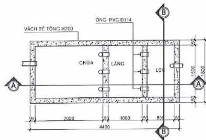
MẶT BẰNG BỐ TRÍ HẠM TỰ HOẠI TỶ LỆ 1/50
