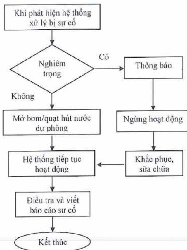
Hình 4-11 Sơ đồ U'PSC hệ thống xử lý khí thải
