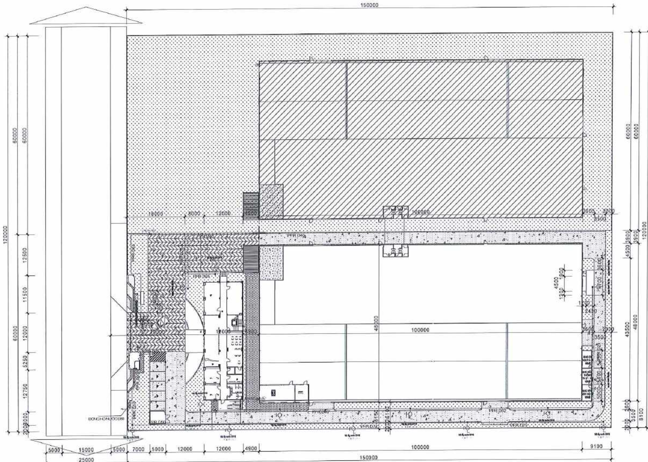
TỔNG MẶT BẰNG CẤP NƯỚC TỶ LỆ 1/500
