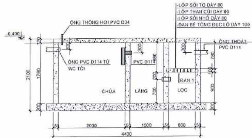
MẶT CẮT A-A TỶ LỆ 1/50
