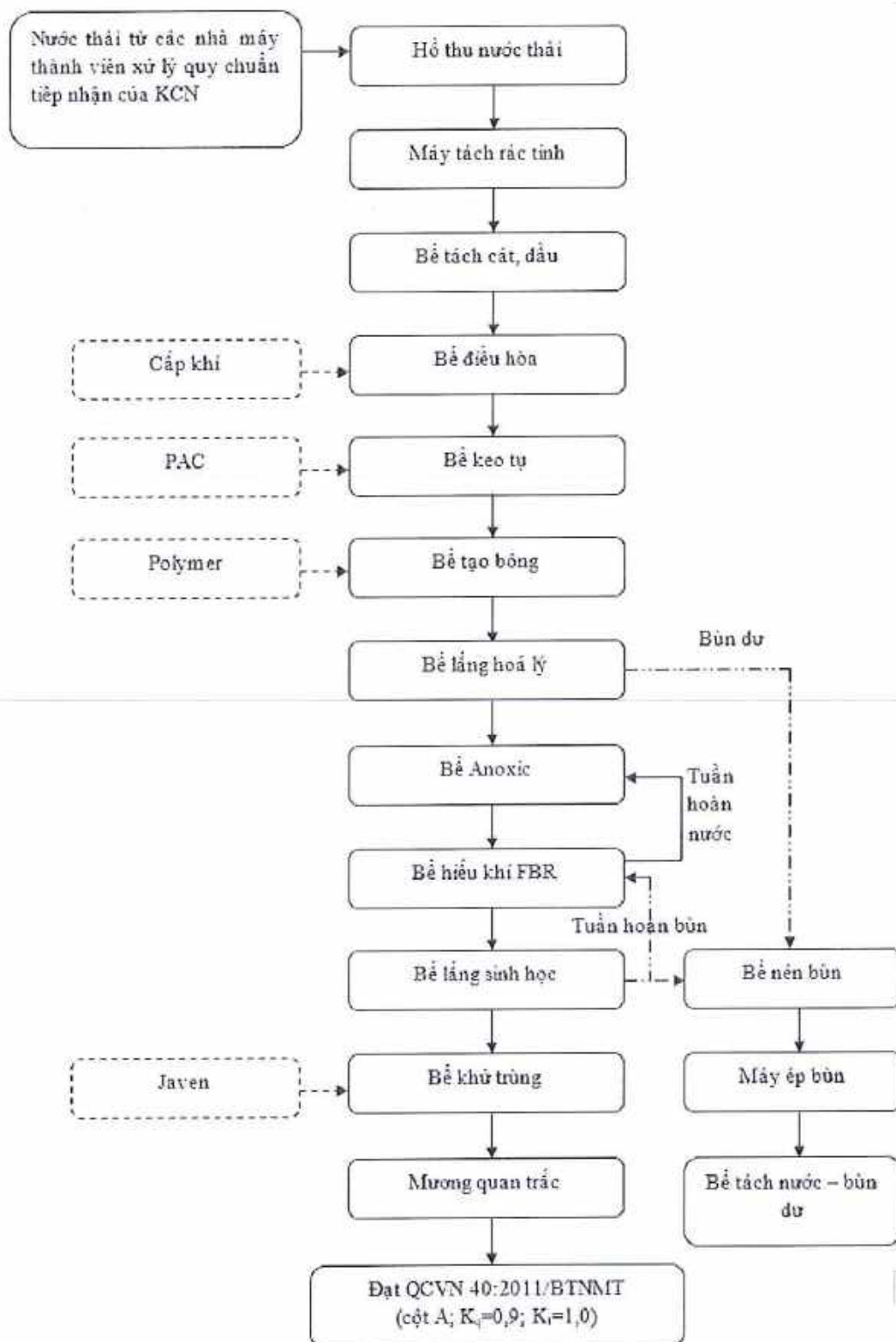
Hình 2-1 Quy trình xử lý nước thải của trạm xử lý nước thải tập trung KCN
