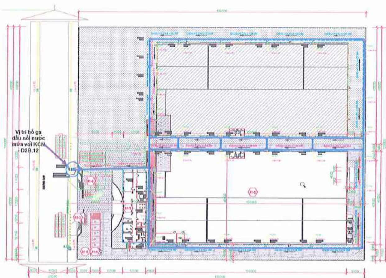
Hình 4-3 Mặt bằng thoát nước mưa
