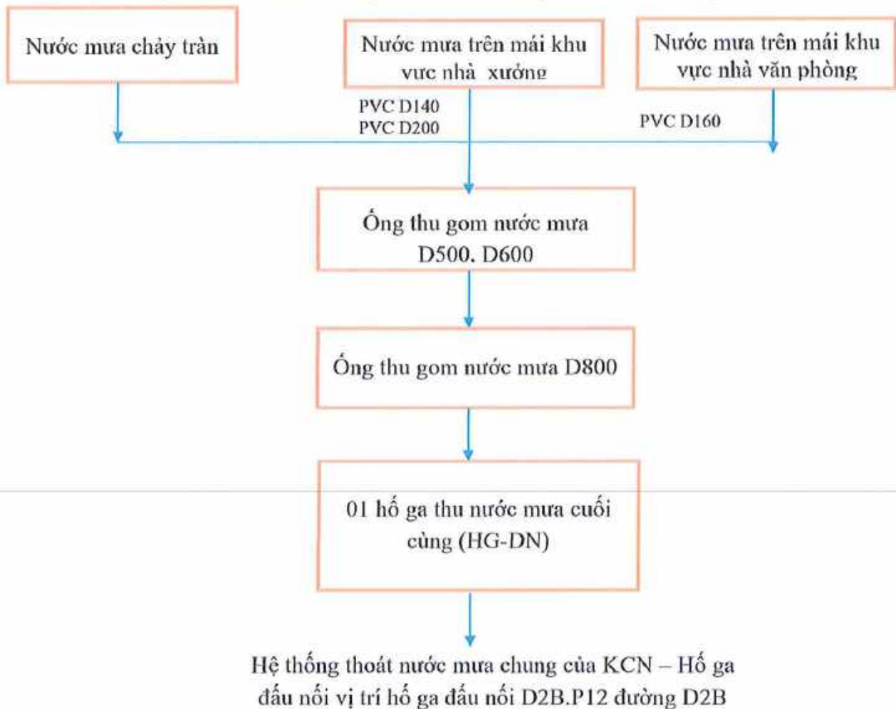
Hình 4-5 Sơ đồ thu gom, thoát nước mưa
