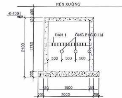
MẶT CẮT B-B TỶ LỆ 1/50
